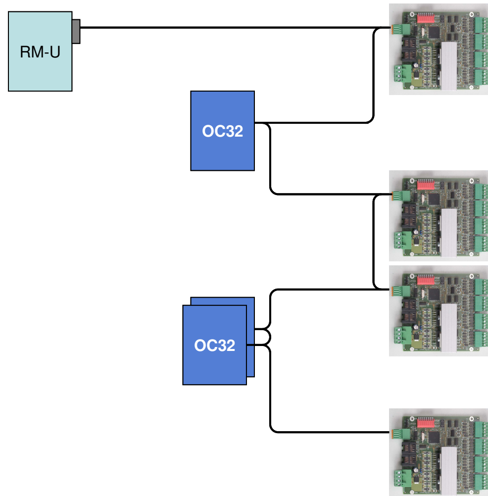
Abb. 13: Netzwerkverkabelung zwischen Dinamo-Modulen, Beispiel Methode 1
