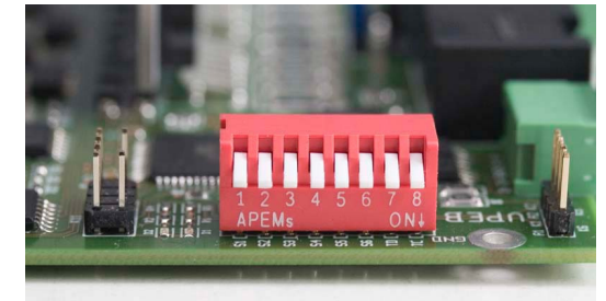
Abb. 15: TM44 DIPschalter
