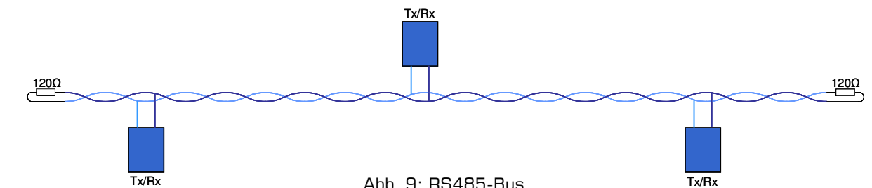
Abb. 9: RS485-Bus
