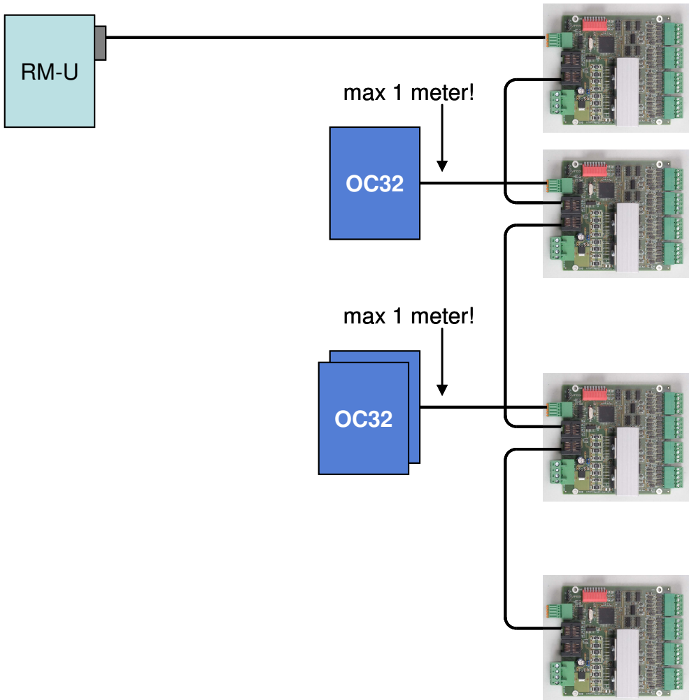
Abb. 14: Netzwerkverkabelung zwischen Dinamo-Modulen, Beispiel Methode 2
