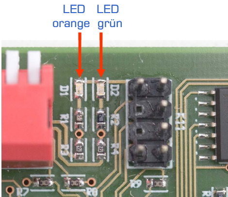
Abb. 16: TM44 LEDs
