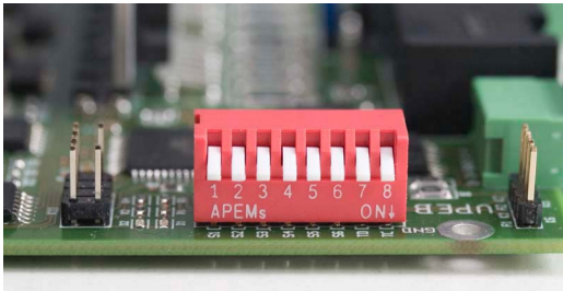
Abb. 12: TM44 DIPschalter
