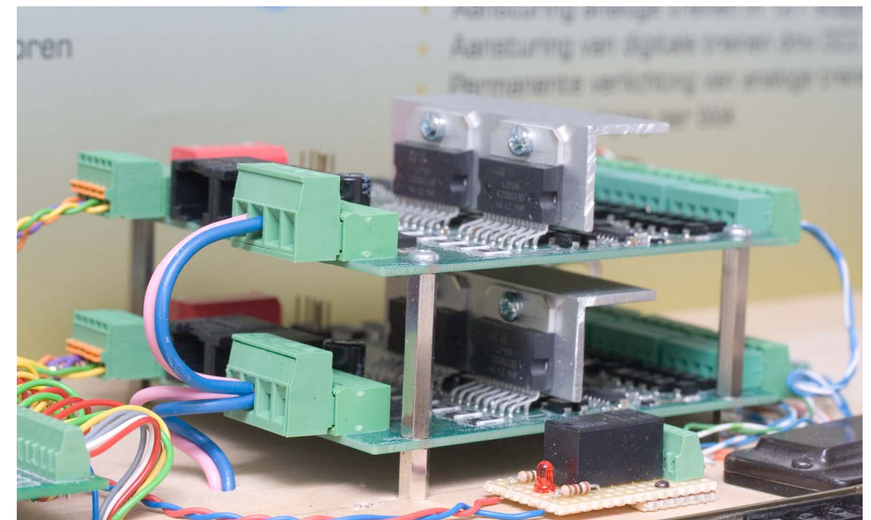
Abb. 3: Montage mehrerer TM44-Module
